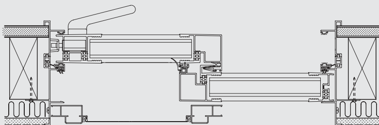
Sliding Door Detail
